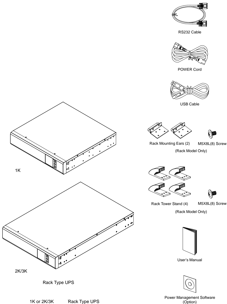
Рис.1. Комплектация
