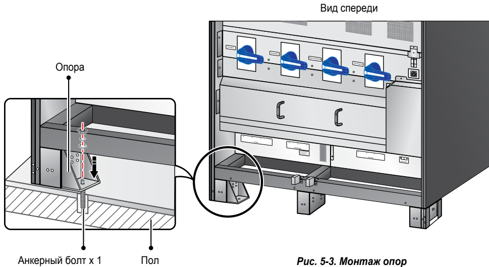
Рис. 5-3. Монтаж опор
