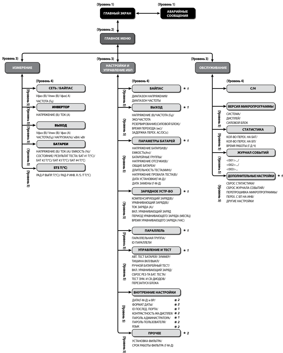
Рис. 8-1. Структура экранных меню
