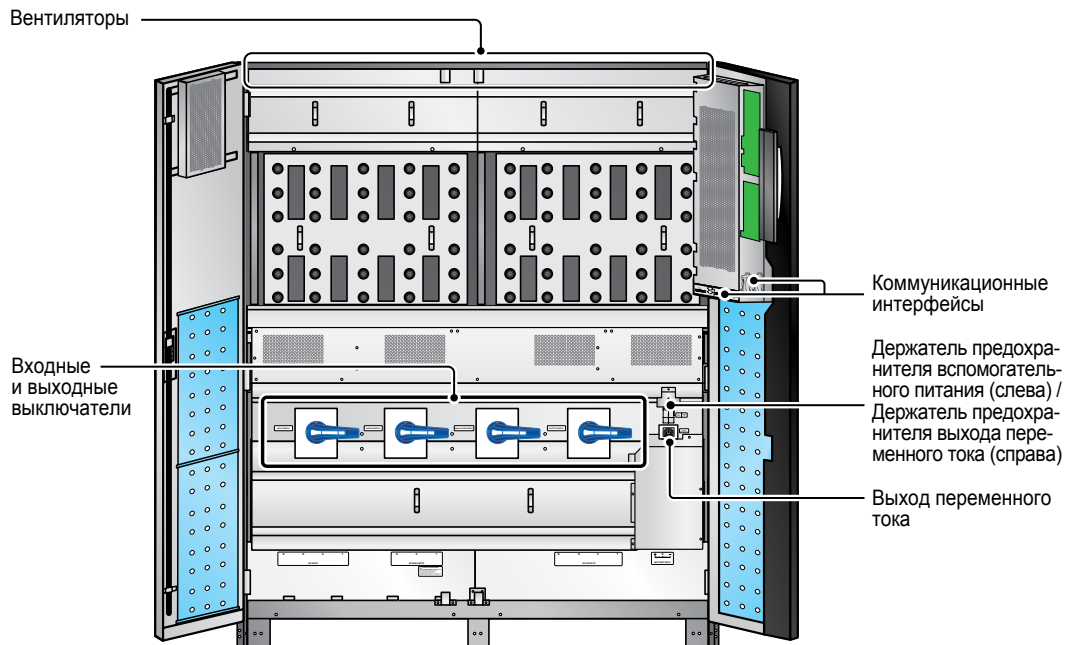
Рис. 2-4. Внутреннее устройство
