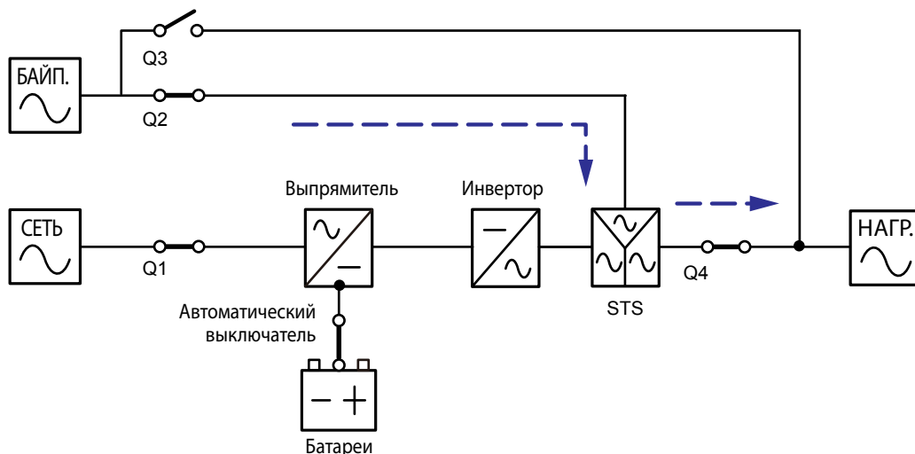
Рис. 3-3. Передача электроэнергии через ИБП в режиме байпаса
