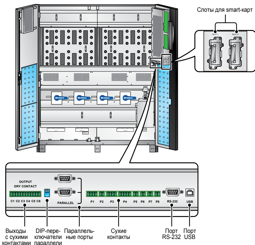
Рис. 4-1. Коммуникационные интерфейсы
