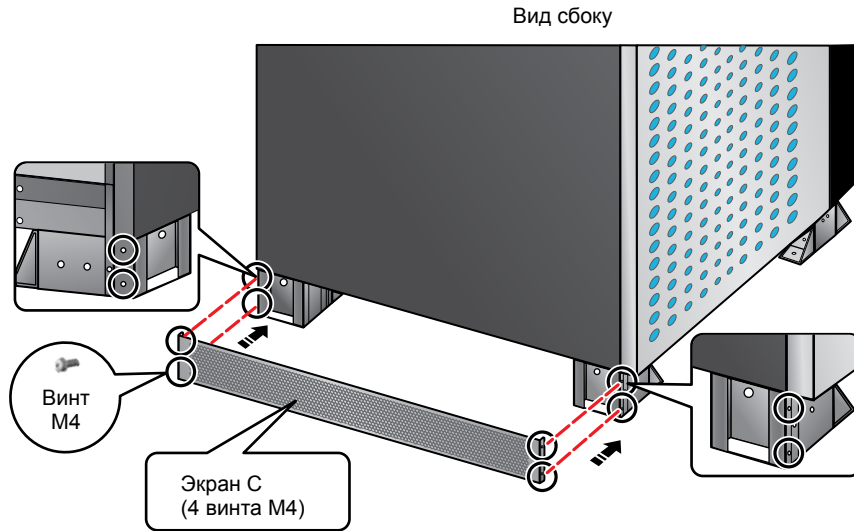
Рис. 5-6. Установка экранов для защиты от грызунов с боковых сторон ИБП
