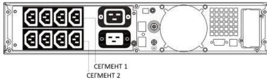
Рисунок 32. 3000 ВА Rack/Tower
