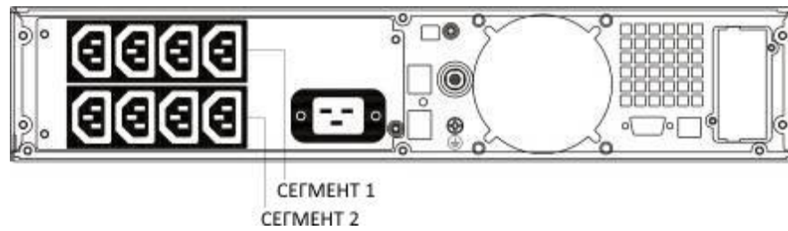
Рисунок 31. 1500/2000 ВА Rack/Tower
