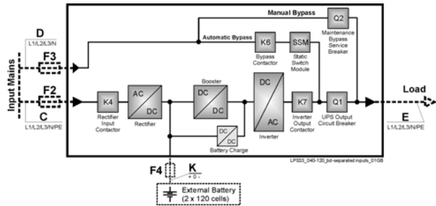
Рис. 4.7.3-2 Раздельные входы Выпрямителя и Байпаса (опция)
