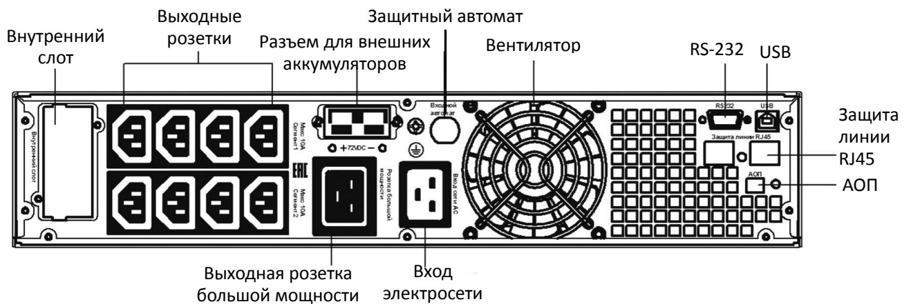
Рис. 3 Задняя панель ИБП мощностью 1.5 кВА, 2 кВА, 3 кВА (розетка C19 только на модели 3 кВА)
