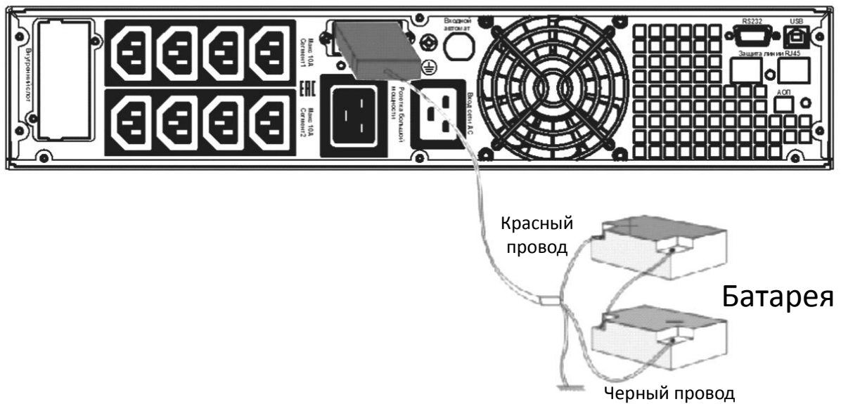
Рис. 7 Подключение внешней аккумуляторной батареи для увеличения времени автономной работы
