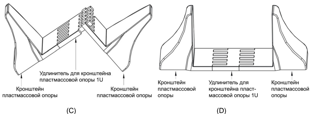
Рис. 9 Пластмассовая опора для ИБП в корпусе высотой 3U
