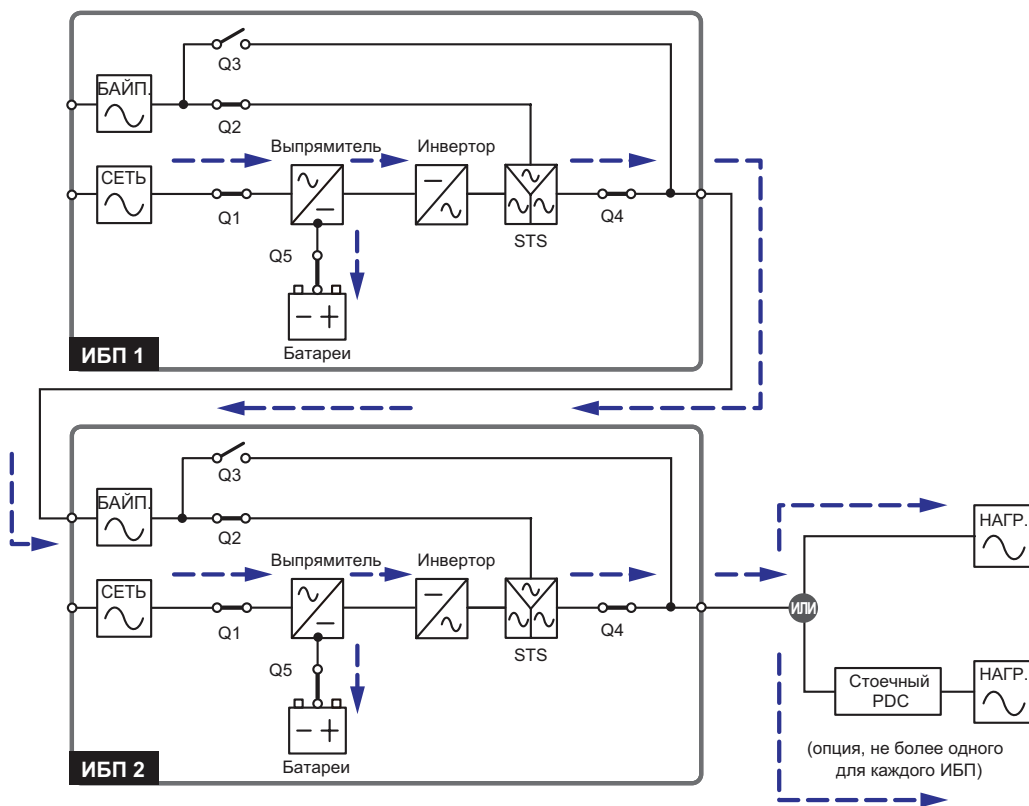
Рис. 3-10. Последовательное резервирование
