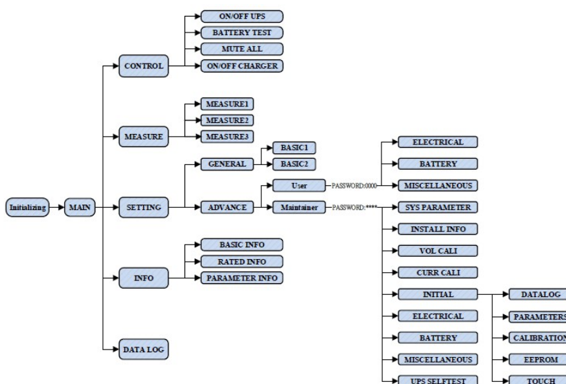
Рисунок 9: Структура меню.
