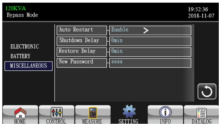
Рисунок 20: Подменю MISCELLANEOUS.
