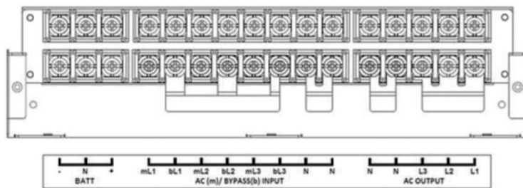
Рисунок 7-5. Установка шины для конфигурации с однофазным выходом и вход от двух источников питания
