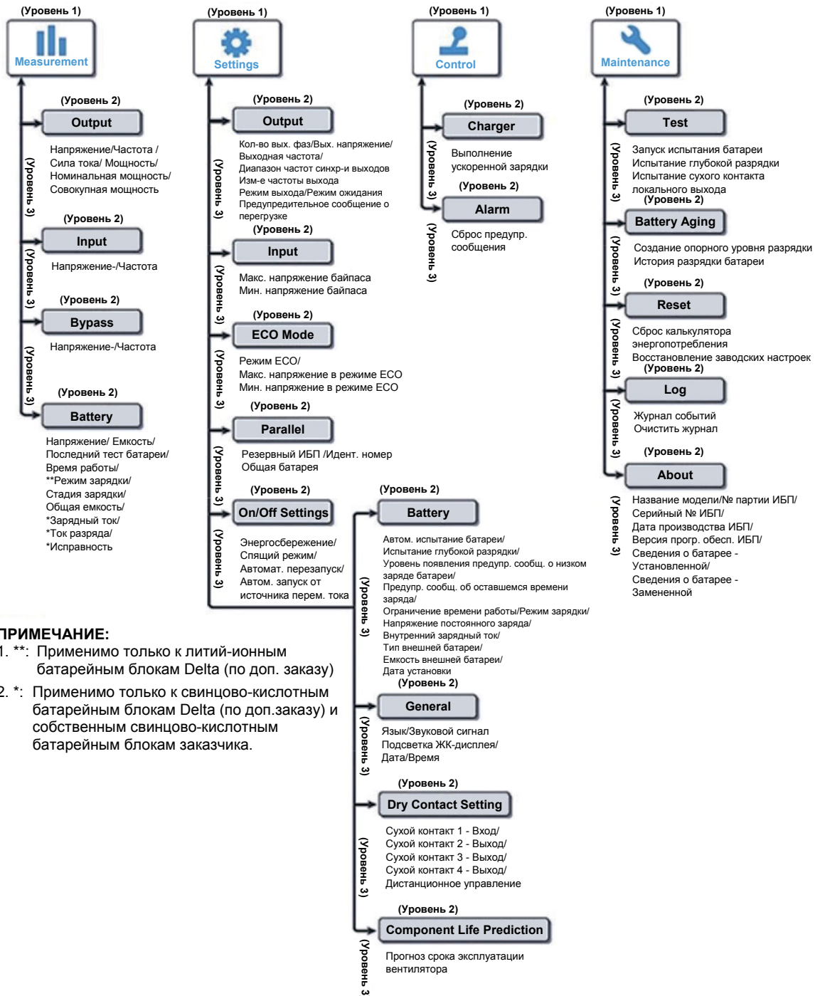
Рисунок 10-1. Дерево меню
