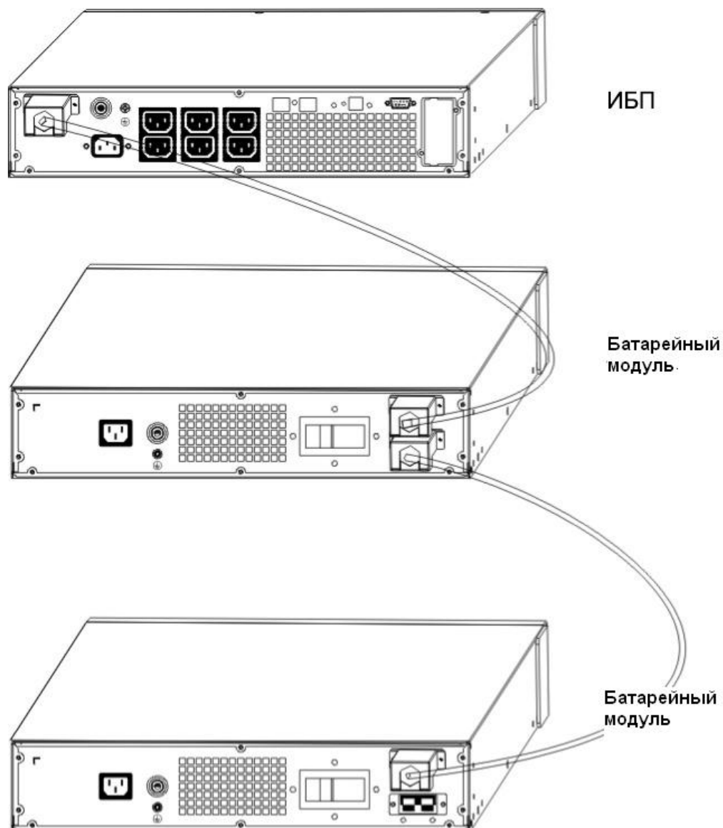
Рисунок 17 Последовательное соединение
