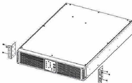
Рис. 3-1. Монтаж ИБП
