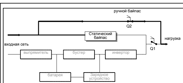
Рис. 4.2-5 Потоки энергии при работе сервисного байпаса
