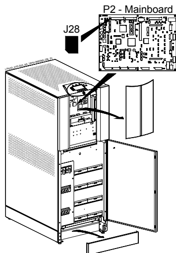
Рис. 10.2.2-4 Основная плата - P2
