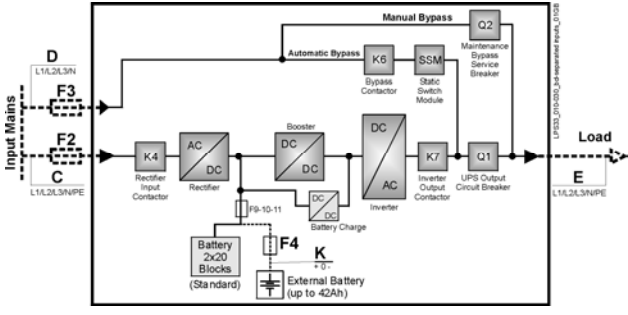
Рис. 5.7.3-2 Раздельный вход выпрямителя и байпаса (опция)
