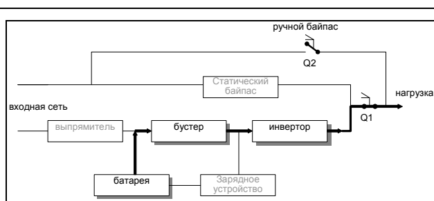
Рис. 4.2-6 Поток энергии при перебое электросети
