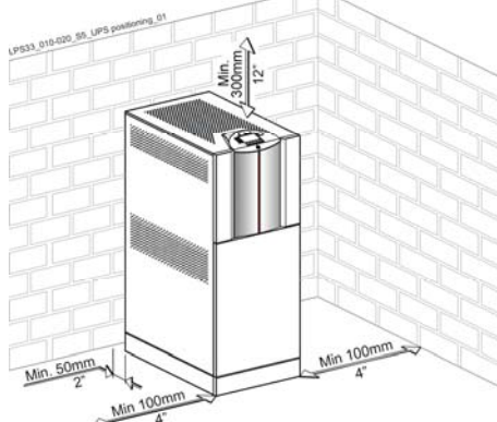
Рис. 5.4-1 Расположение ИБП
