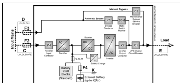
Рис. 5.8.2-1 Раздельный вход выпрямителя и байпаса
