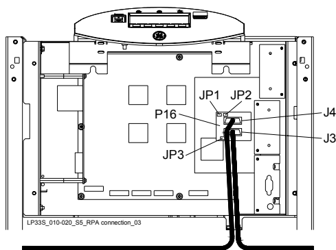
Рис. 5.8.4-3 Подключение к плате P16
