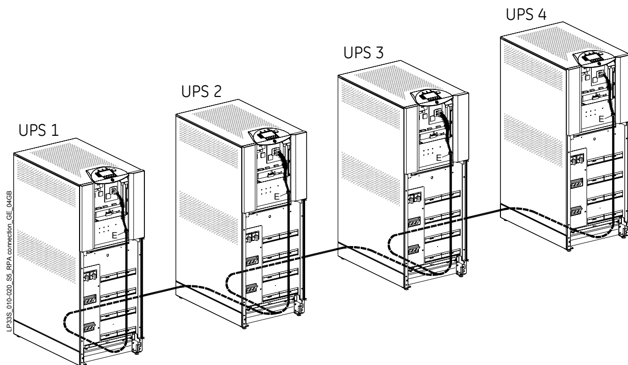
Рис. 5.8.4-4 Расположение параллельной системы RPA
