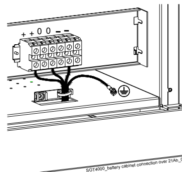
Рис. 10.2.2-3 Батарейный клеммник свыше 21Ah
