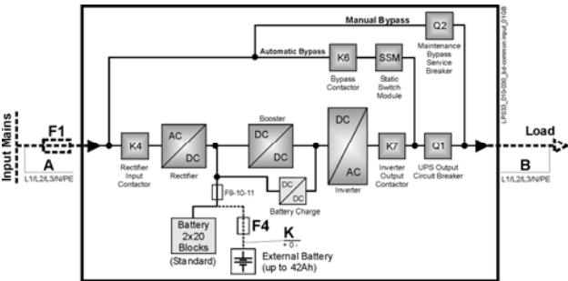
Рис. 5.7.2-2 Общий вход выпрямителя и байпаса
