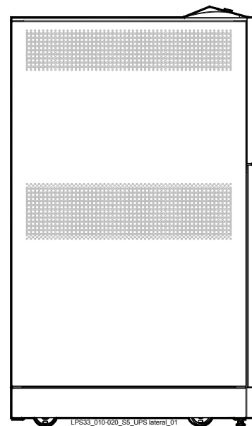
Рис. 2.2-3 Вид сбоку
