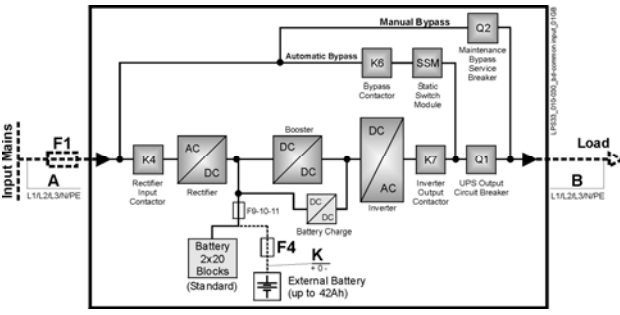
Рис. 5.7.3-1 Общий вход выпрямителя и байпаса
