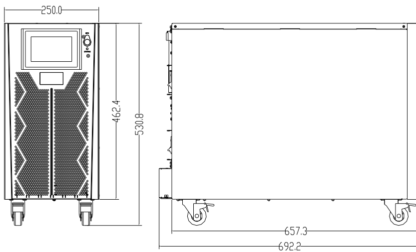
Рисунок 1-1 Размеры ИБП 10/15 kVA (стандартный типоразмер)
