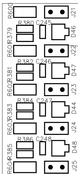
Рисунок 5-12 Плата контроля (PS1203_CT1)
