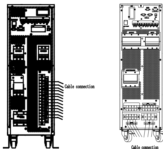
Рисунок.3-10 Кабельные вводы
