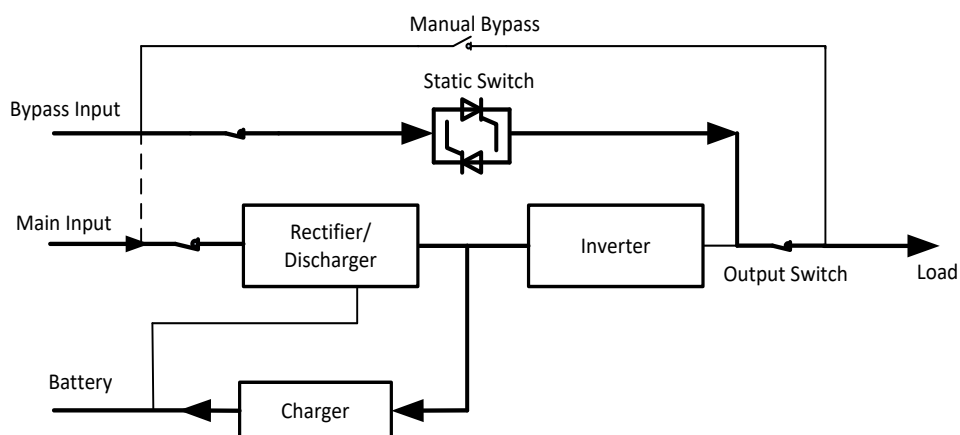
Рисунок.2-6 Режим ESO
