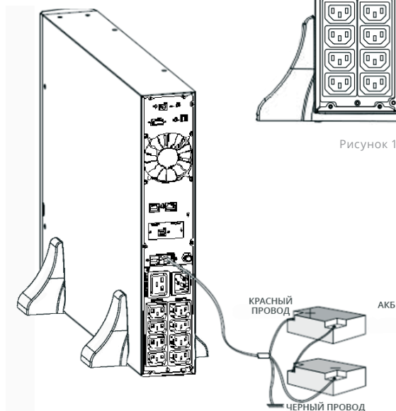
Рисунок 12. Подключение ВБМ
