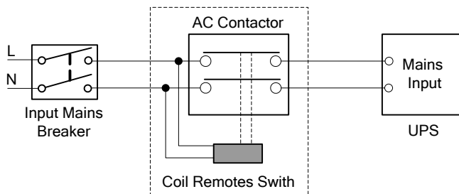
Рис.4-1 Типовая установка внешнего изолирующего устройства
