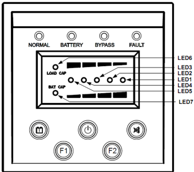
Рис.5-1 Светодиодная панель
